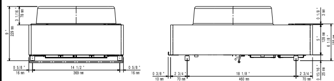
Oldalnézet
